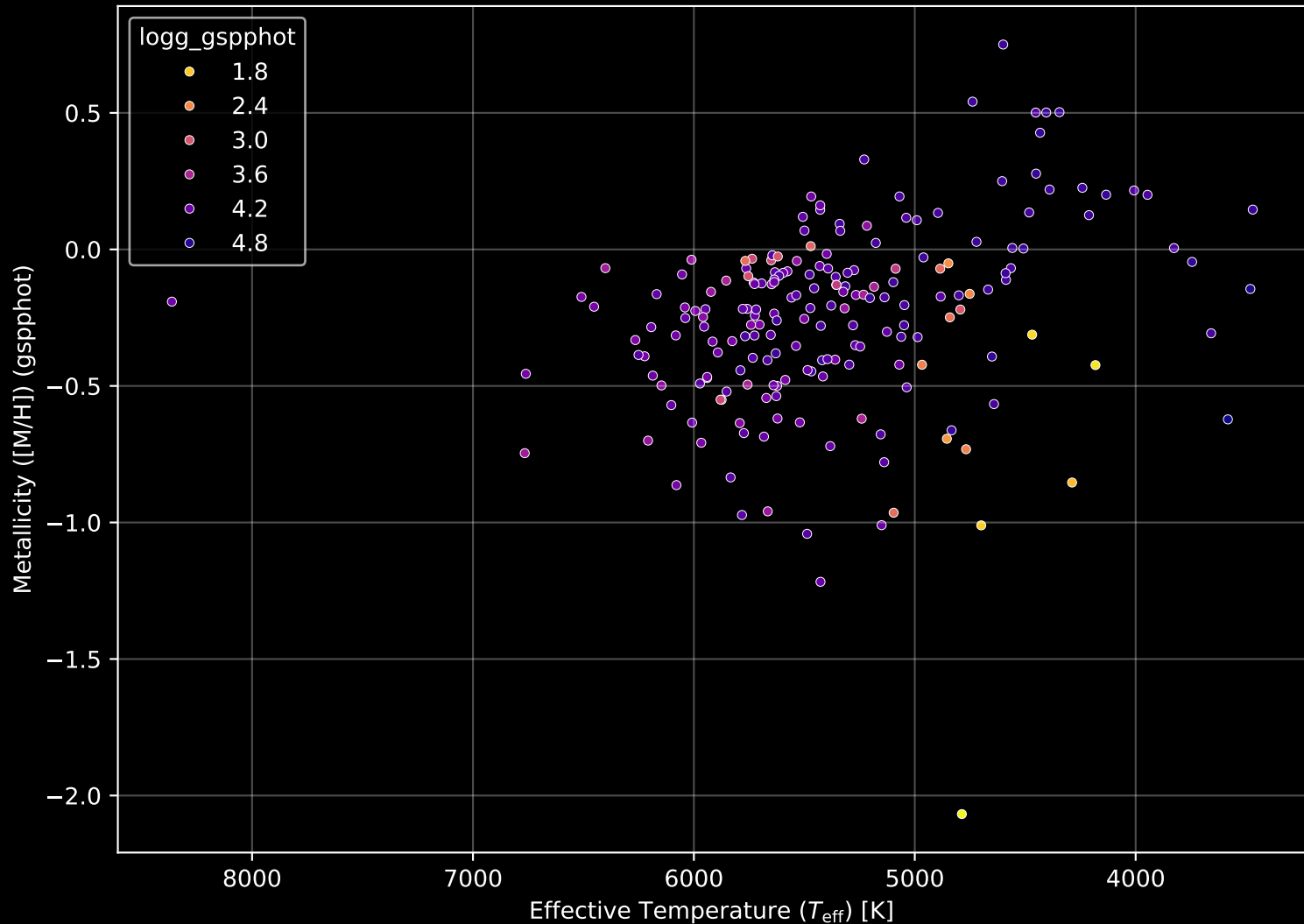
APOGEE DR17 Field: [046-47-O] Stellar Population Parameters (n= 199)
